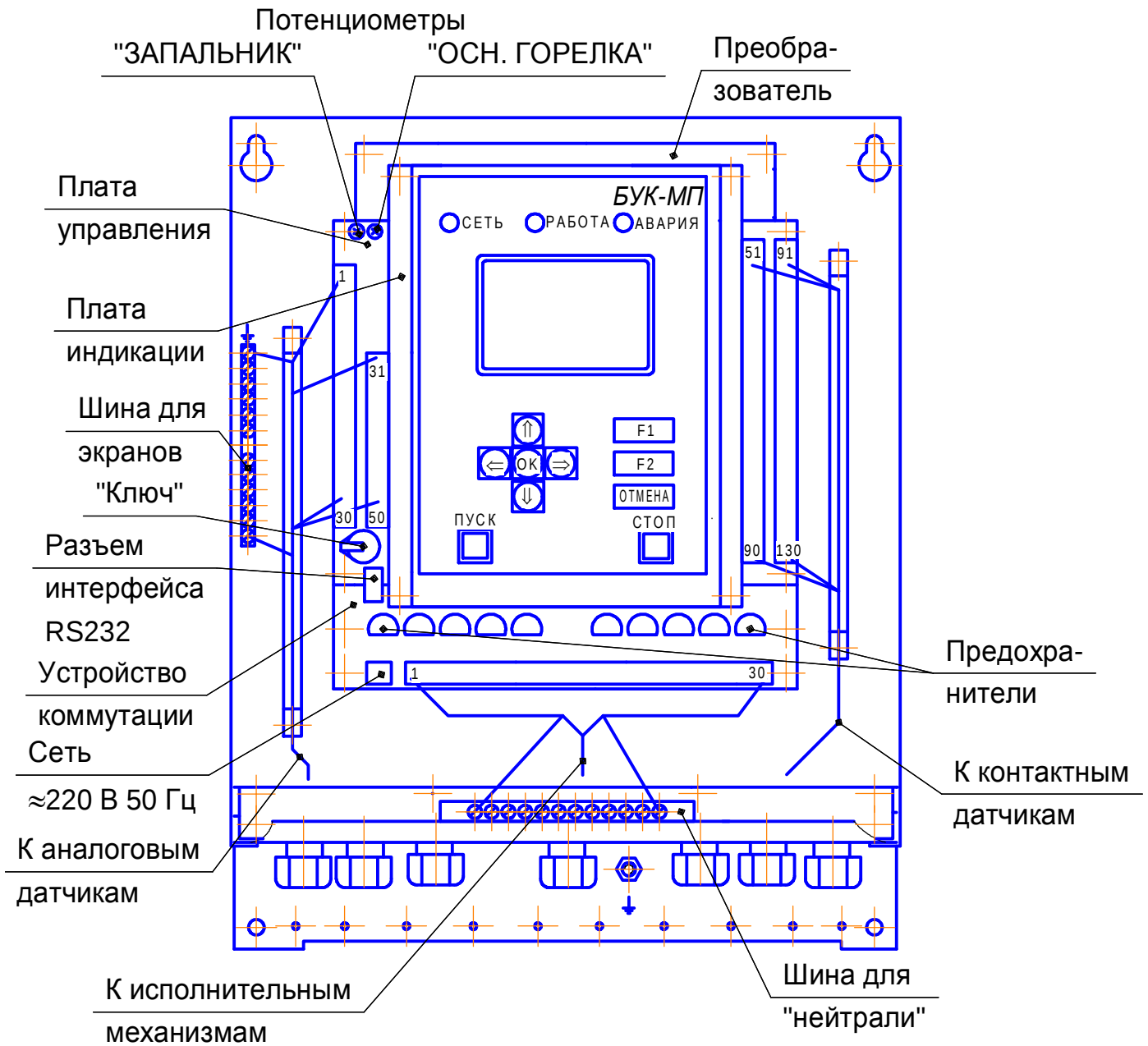
Рис. 2. Расположение разъемов на платах.
