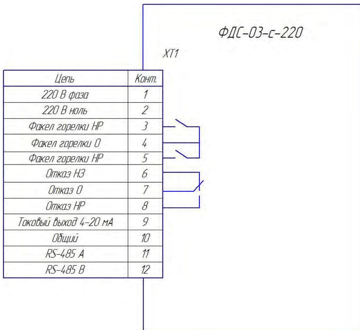
Рис.4 Схема подключения внешних цепей
