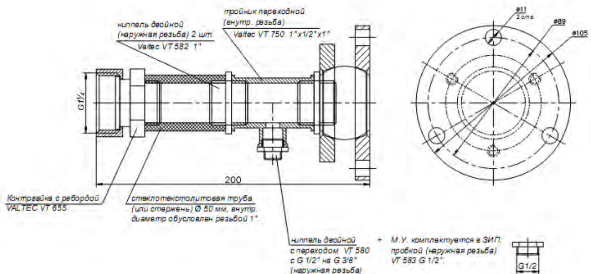
Рис.5б. Монтажный узел юстировочный CE-07-05.
