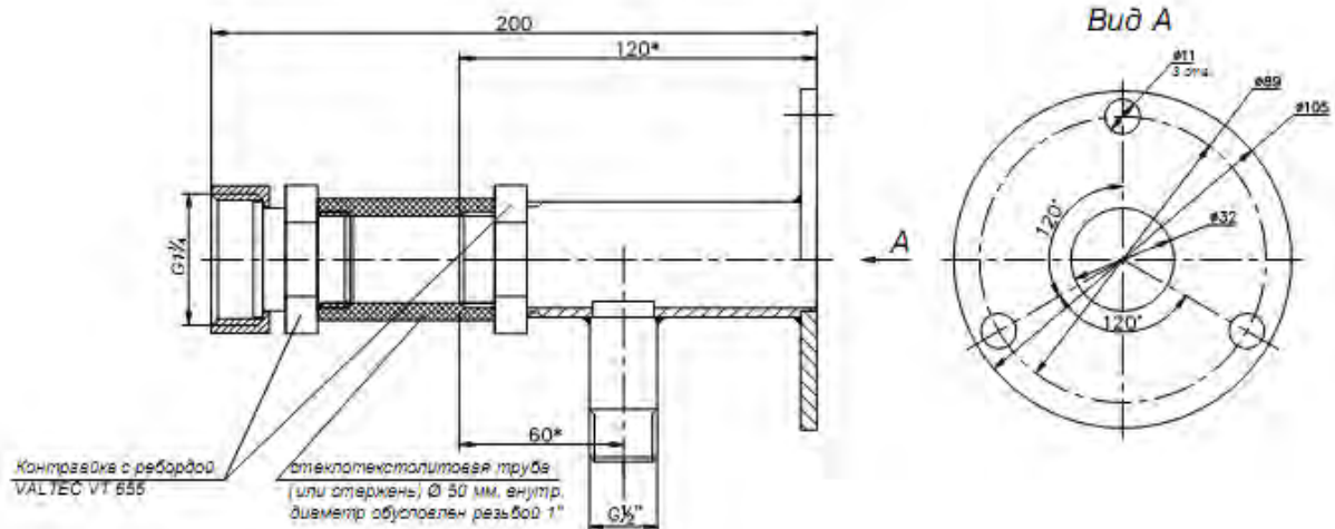
Рис.5а. Монтажный узел CE-07-06.
