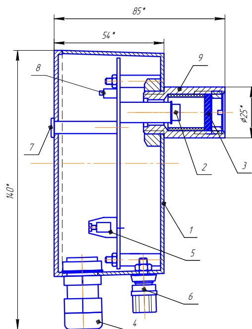
Рис.2 Конструкция фотодатчика
