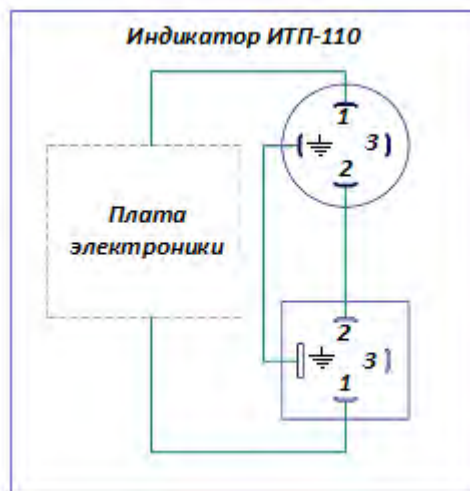
Рис.4. Маркировка контактов соединителей DIN 43650.
