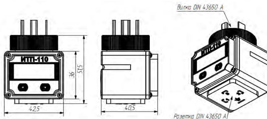
Рис.1. Общий вид и габариты ИТП-110.
