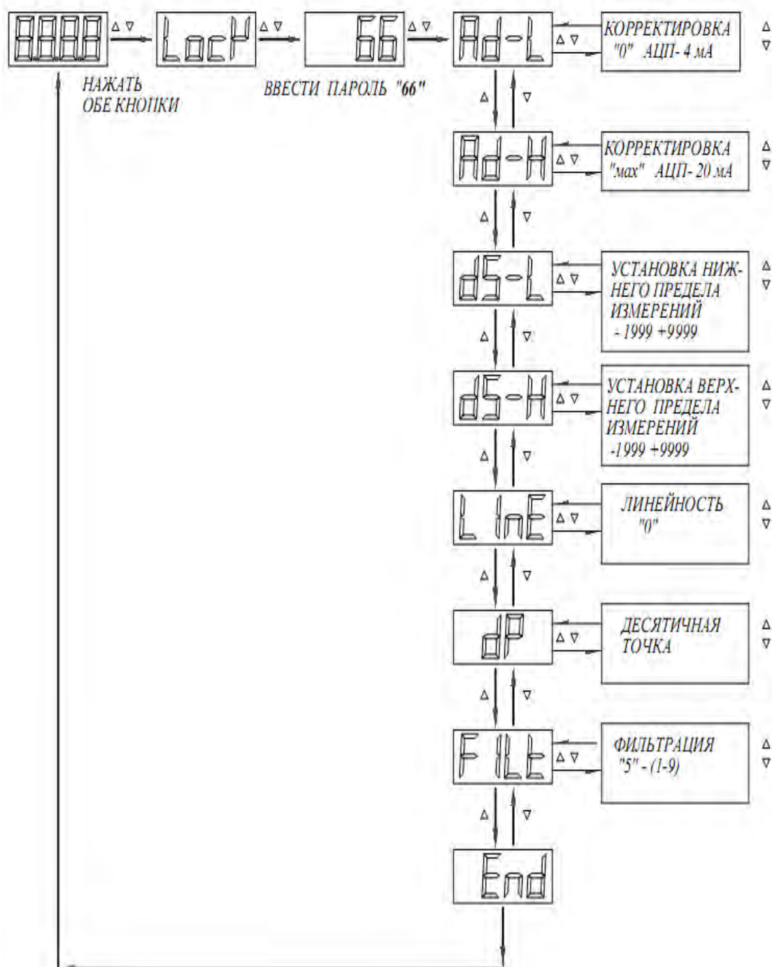
Блок-схема настройки ИТП-110
