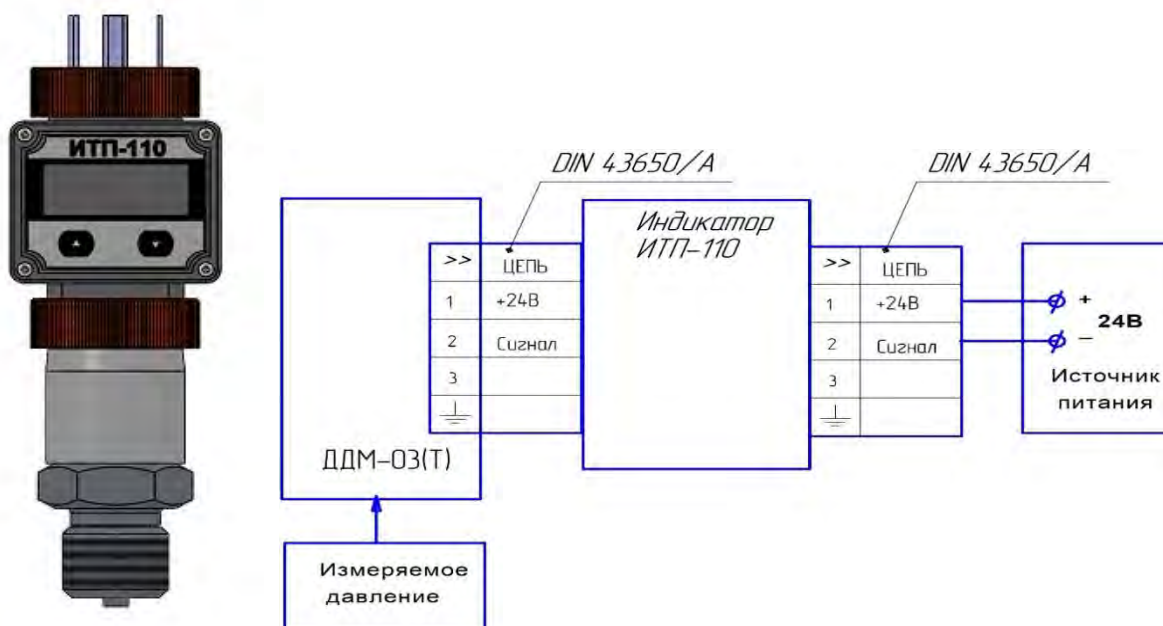
Рис.3. Пример монтажа на датчик давления ДДМ-03Т.
