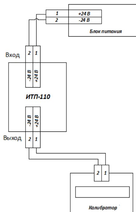
Рис.5. Схема калибровки АЦП ИТП-110.
