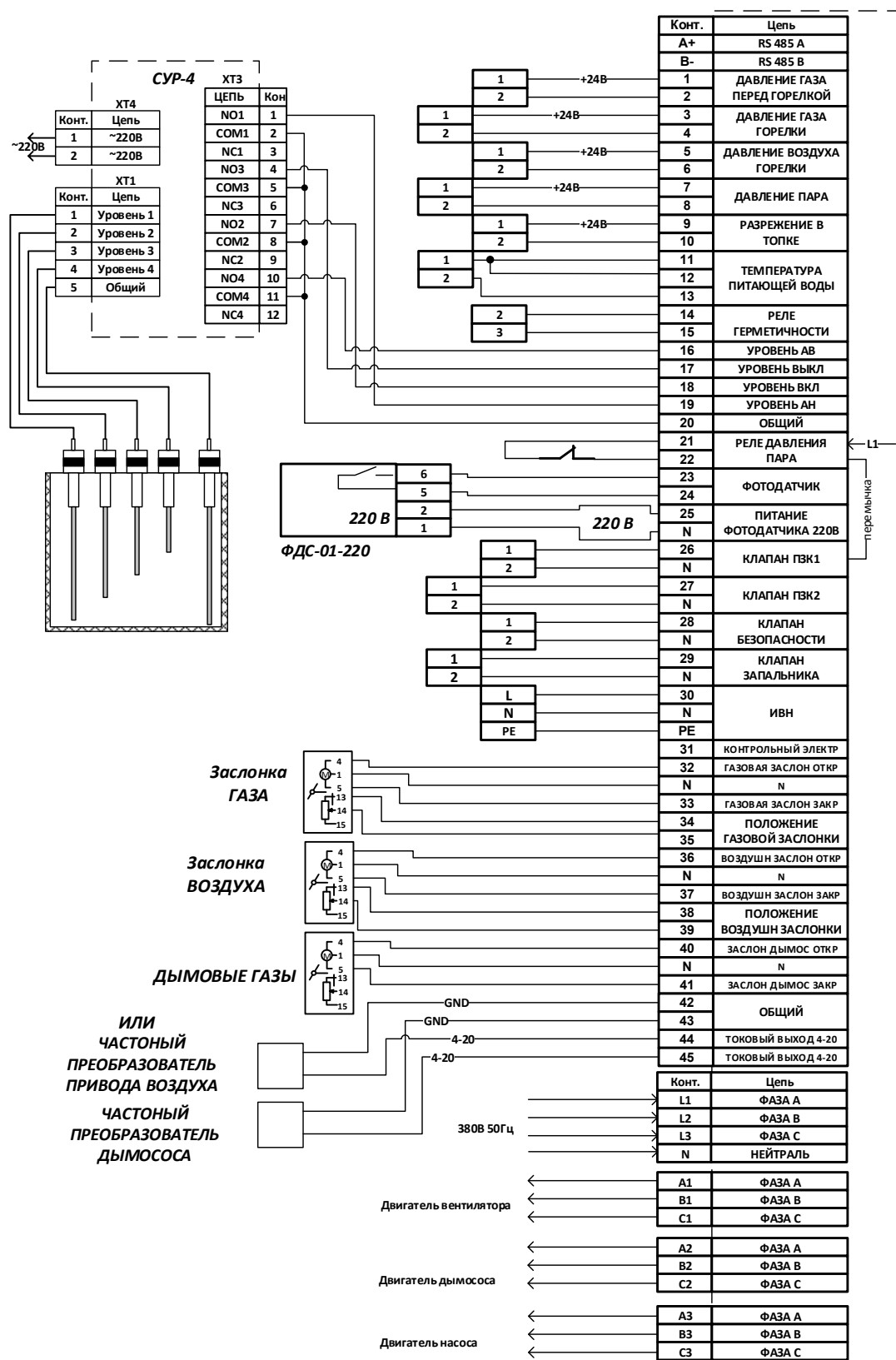
Рис. 5: Клеммник шкафа.
