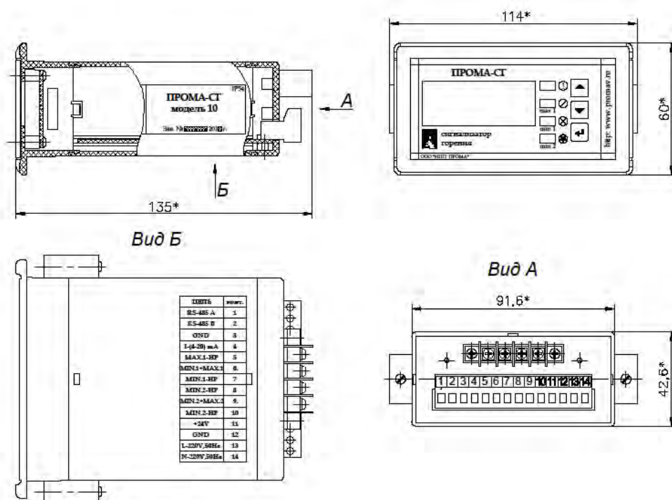
Рис.24а. ПРОМА-СГ-Щ щитовой
