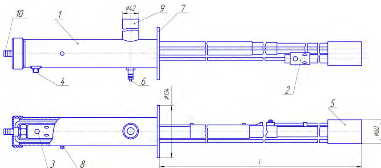
Рис. 10. Общий вид запальной горелки ЗГИ- 1/5Б.
