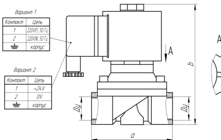
Рис. 17. Клапан электромагнитный КЭГ-15.
