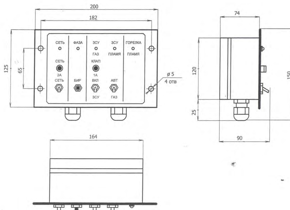
Рис.34а. Местный щит управления МЩУ. Общий вид.
