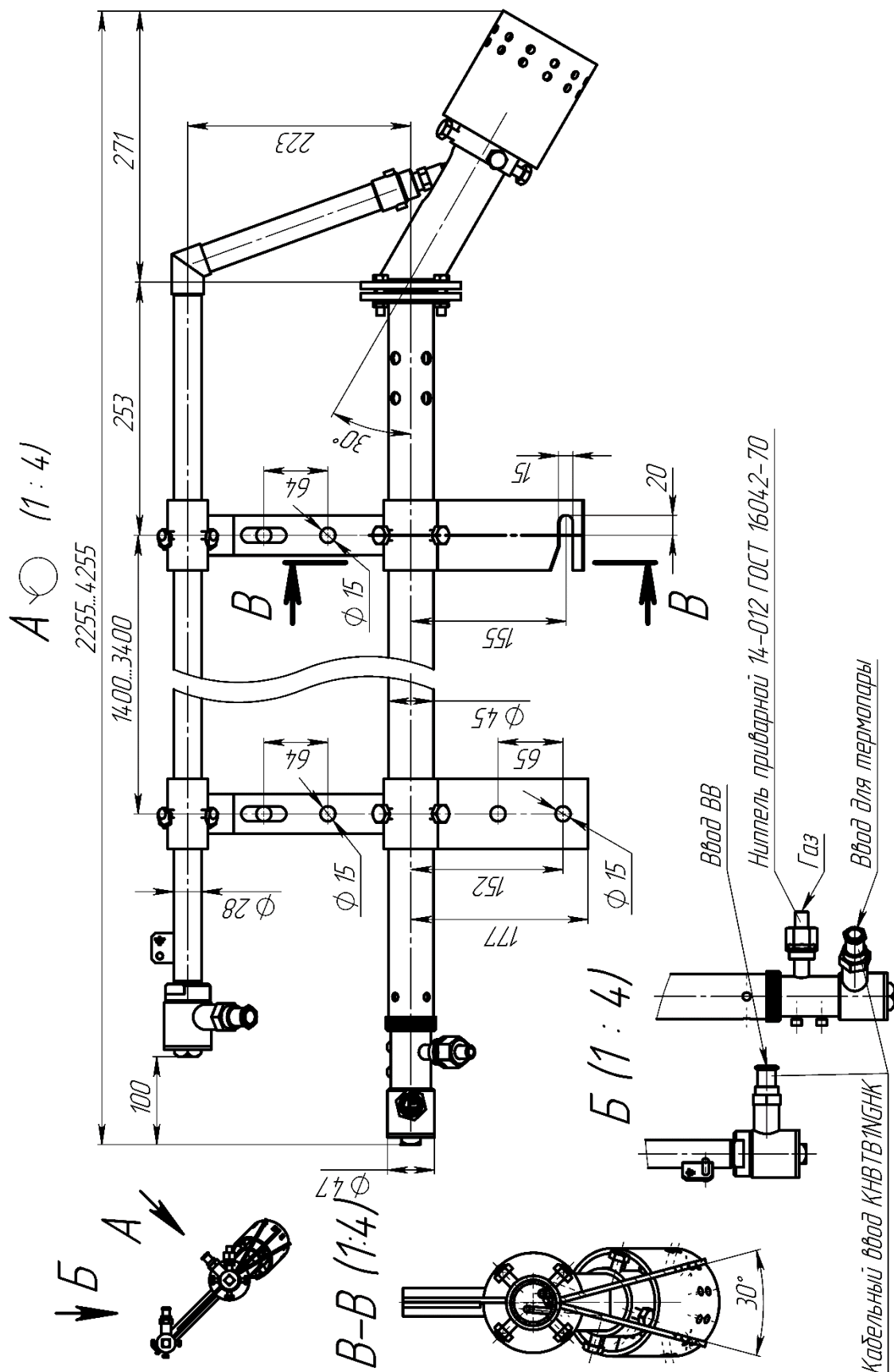
Рис.8. Общий вид запальной (пилотной) горелки ЗГИ-45-ФС с диаметром ствола 45 мм с электроискровым розжигом и контролем факела запальной горелки термопарой.
