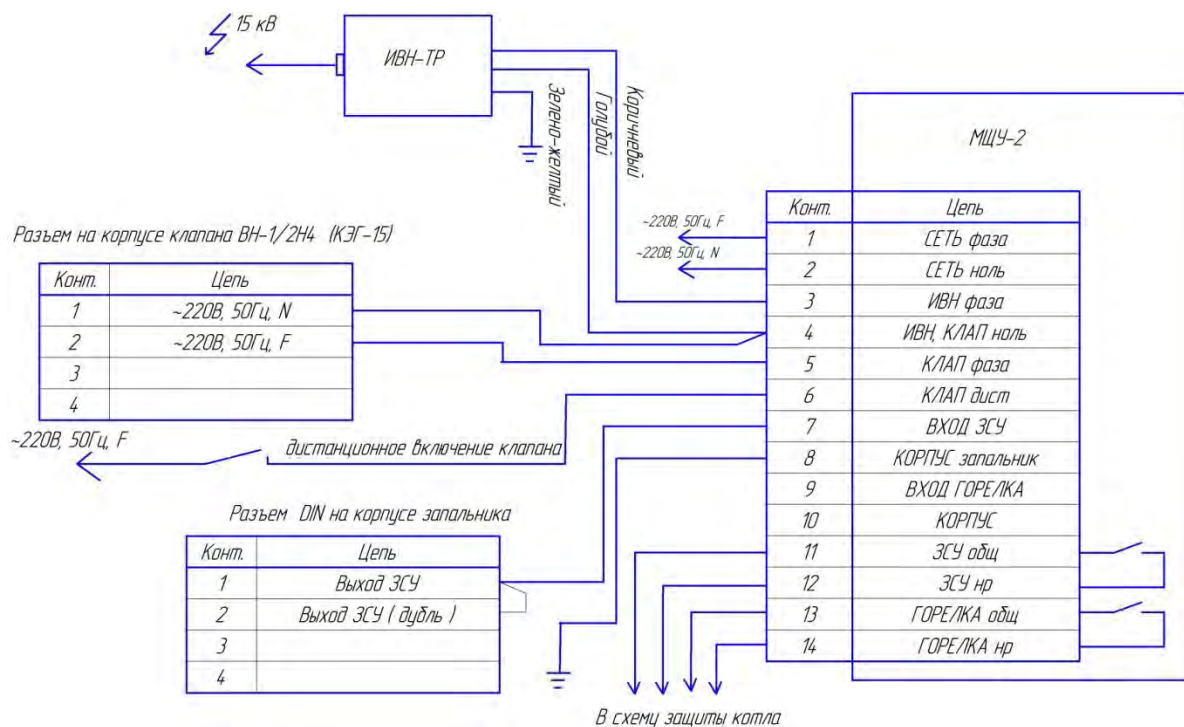
Рис.346. Местный щит управления МЩУ-2. Схема подключения.
