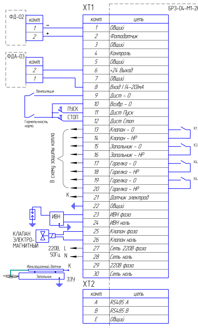
Рис.33. Схема внешних подключений блока розжига запальника БРЗ-04-М1-2К.
