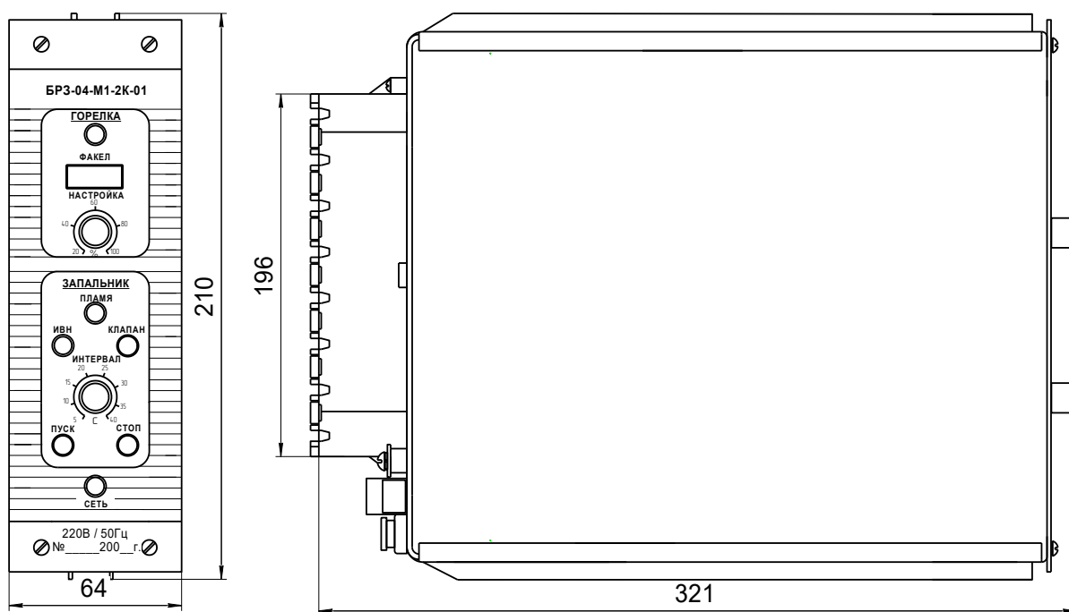
щитовое исполнение
