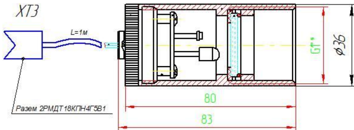
Габаритные размеры устройства контроля пламени ФДСА-03М – 05.
