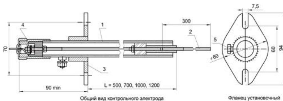
1-ствол, 2 –электрод жаропрочный, 3 –фланец, 4 –кожух, 5 –винт стопорный
